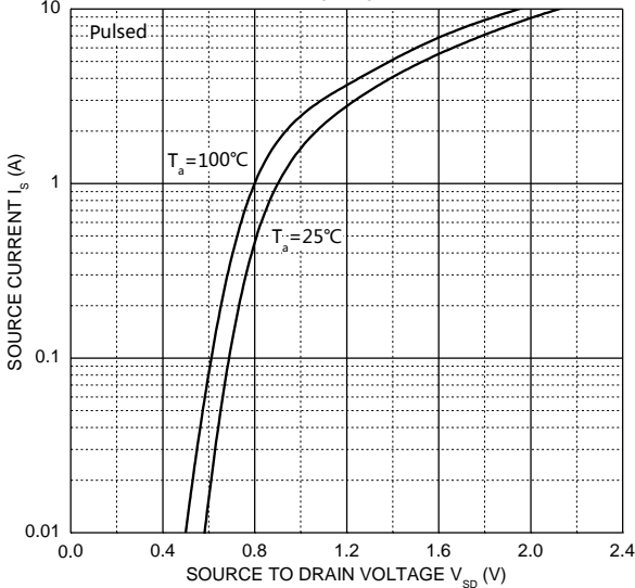
I_S - V_{SD}
