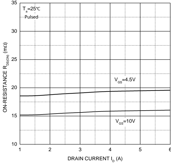
R_{DS(ON)} - I_D
