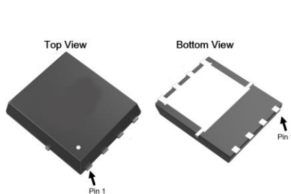
PDFN5X6-8L
