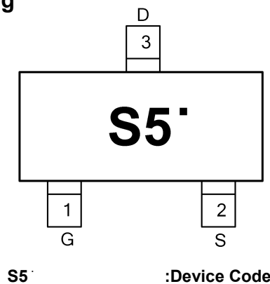
SOT-23
