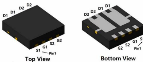
PDFN3X3-8L
